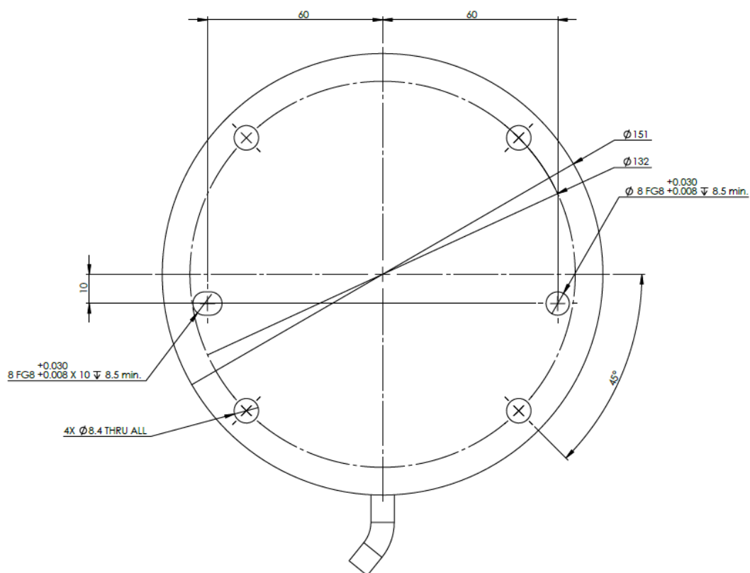
1.1: 机器人基座的底部视图
